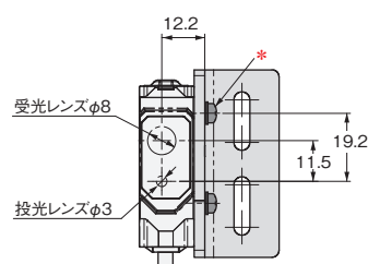
センサ装着時の寸法 (例: 形E3AS-HL500□)
