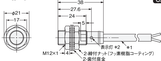
形E2EQ-X3D1
