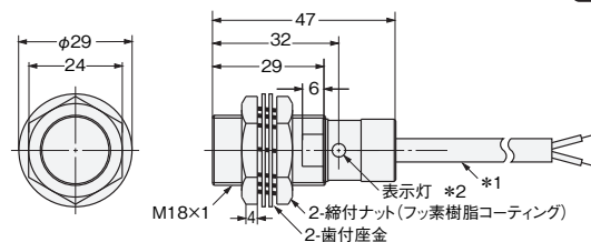
形E2EQ-X7D1
