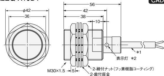
形E2EQ-X10D1
