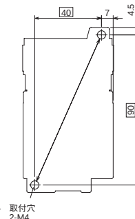
取付穴寸法図
