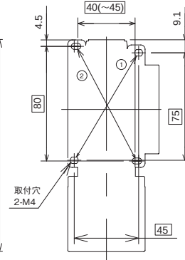
取付穴寸法図
