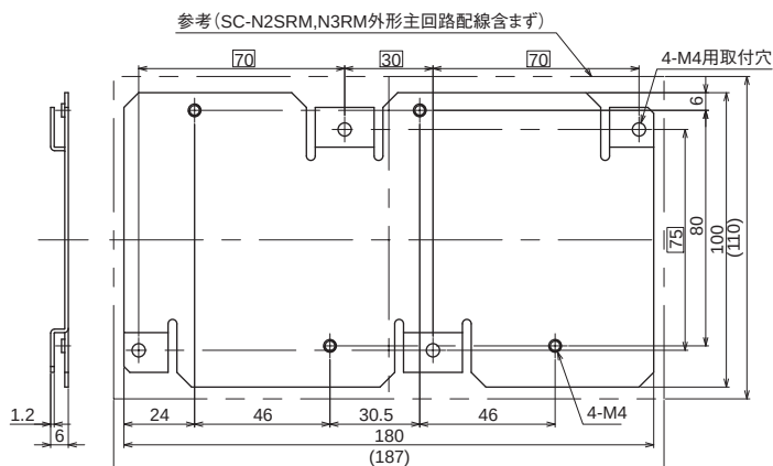
SZ3APR50X形
