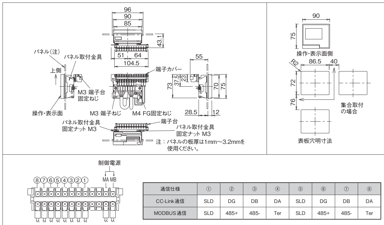
パネル表示ユニットの外形図
